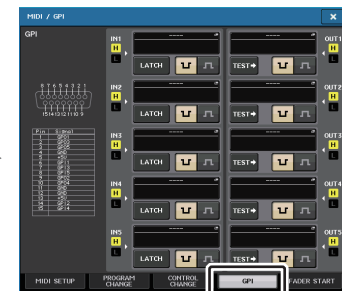
MIDI/GPI 画面
